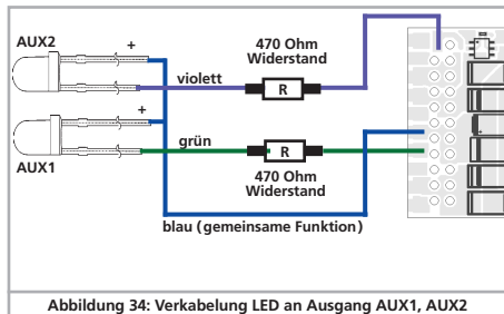
Abbildung 34: Verkabelung LED an Ausgang AUX1, AUX2
