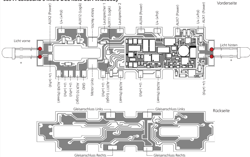
Abbildung 16: LokSound 5 micro DCC Kato USA Widebody
