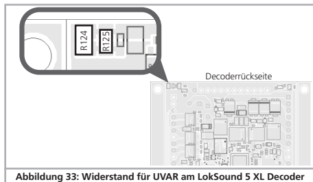
Abbildung 33: Widerstand für UVAR am LokSound 5 XL Decoder
