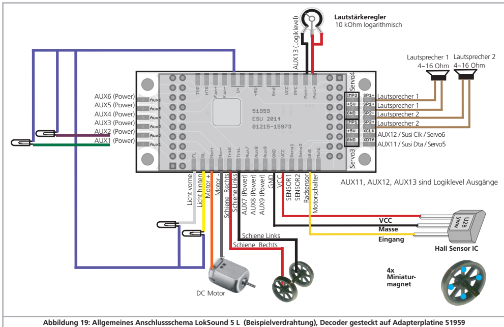
Abbildung 19: Allgemeines Anschlussschema LokSound 5 L. (Beispielverdrahtung), Decoder gesteckt auf Adapterplatine 51959
