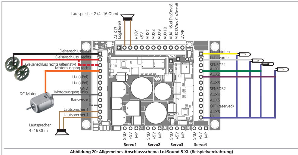
Abbildung 20: Allgemeines Anschlussschema LokSound 5 XL (Beispielverdrahtung)
