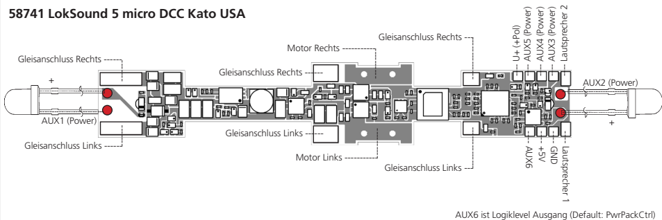
Abbildung 11: LokSound 5 micro DCC Kato USA
