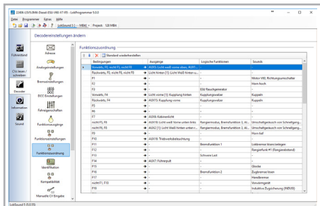
Abbildung 47: Screenshot LokProgrammer, Function mapping
