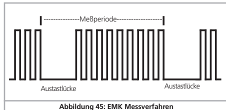
Abbildung 45: EMK Messverfahren
