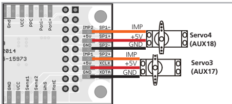
Abbildung 35: RC-Servos an LokSound 5 L
