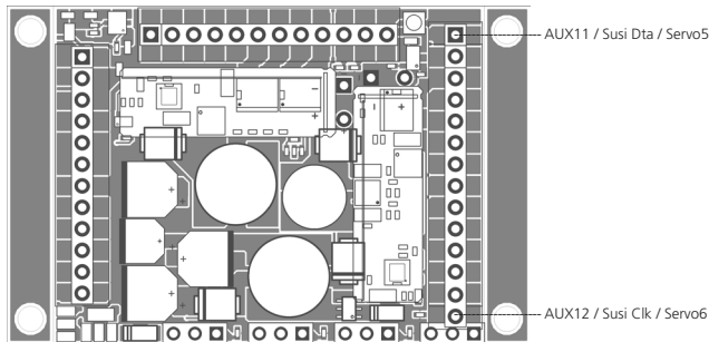
Abbildung 24: LokSound 5 XL Decoder mit Stiftleisten - SUSI Pins für Märklin Lokomotiven
