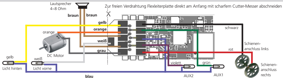
Abbildung 18: Allgemeines Anschlussschema LokSound 5 micro (Beispielverdrahtung, freie Verdrahtung)
