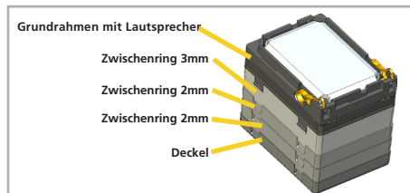
Abbildung 26: Lautsprecher 11x15mm mit Zwischenringen montiert
