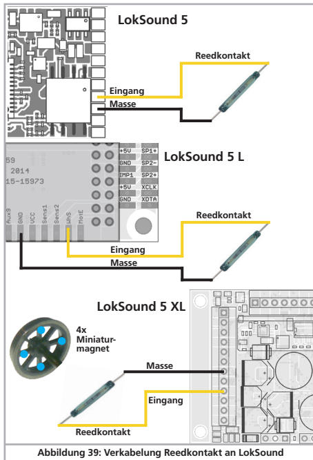
Abbildung 39: Verkabelung Reedkontakt an LokSound
