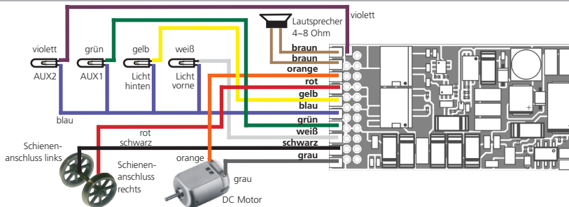
Abbildung 17: Allgemeines Anschlussschema LokSound 5 (Beispielverdrahtung)
