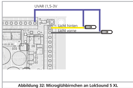
Abbildung 32: Microglühlampen an LokSound 5 XL
