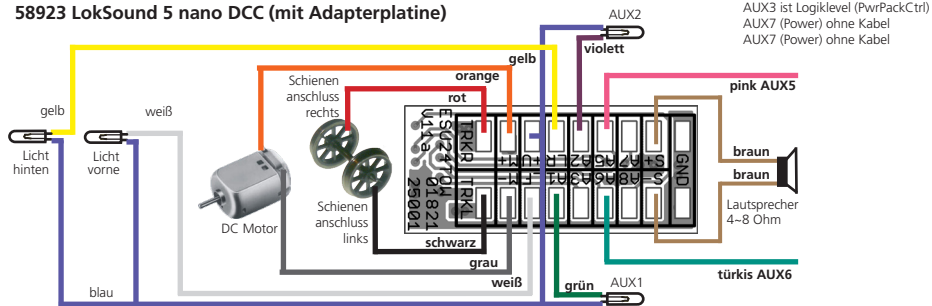
Abbildung 13: LokSound 5 nano DCC
